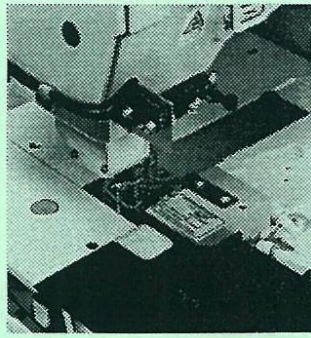
▲ エア式ヘムフォルダーと上送り機構 (写真上)
