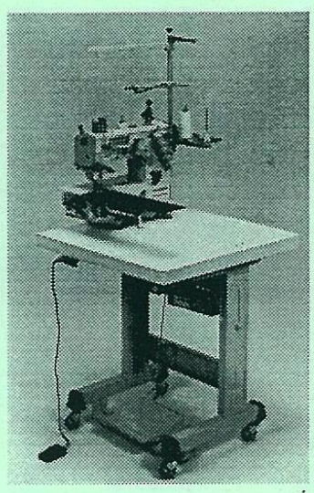
▲ エア式ヘムフォルダーと上送り機構 (写真上)
