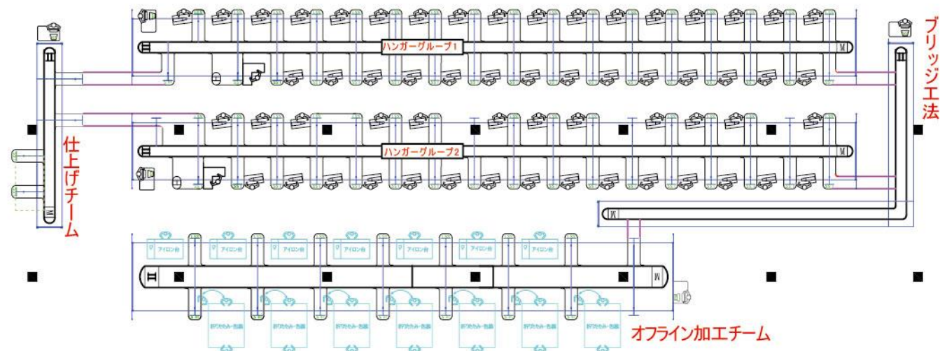
スーツ製造工場レイアウト図
