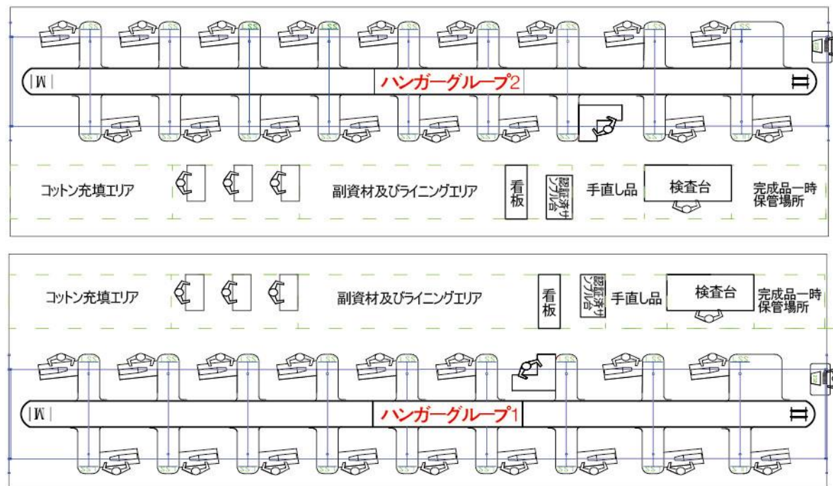
魚釣りバッグ製造工場レイアウト図
