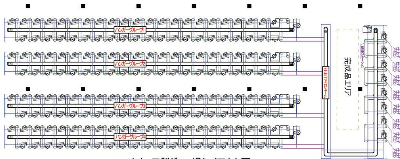
ニットウェア製造工場レイアウト図
